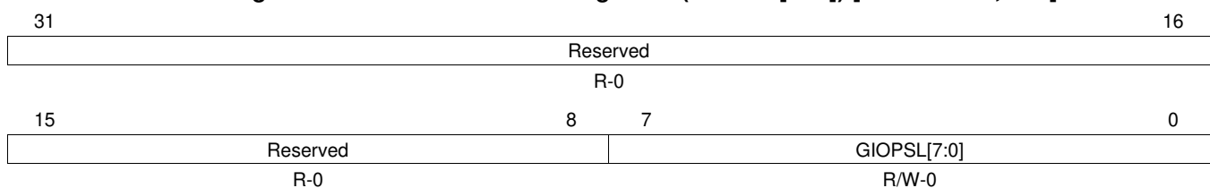
Figure 22-24. GIO Pull Select Registers (GIOPSL[A-B]) [offset = 50h, 70h]
